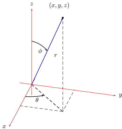
Schema der Kugelkoordinaten in R^3 .
